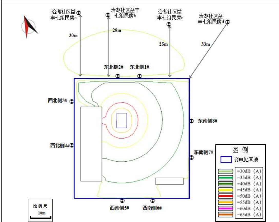
图 6 益丰 110kV 变电站本期工程噪声预测等值线图
