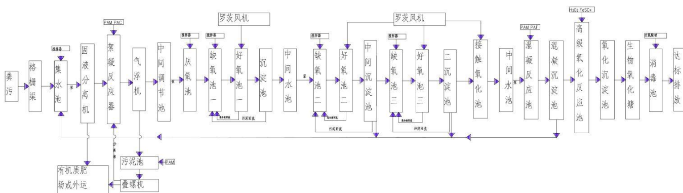
图 4.4-1 项目污水处理工艺流程图
