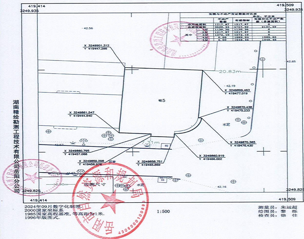
张建秀太阳桥建材大市场内违法建设(4栋)现状审批图
